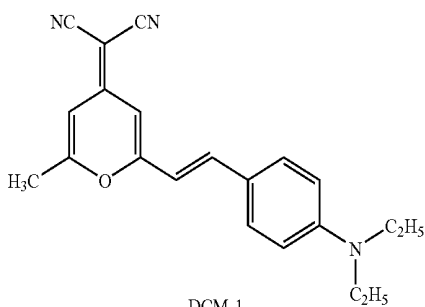
DCM-1
